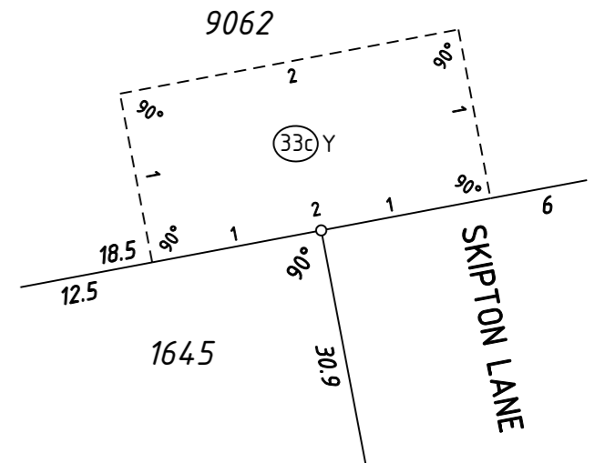
ENLARGEMENT 'D' SCALE 1:40
