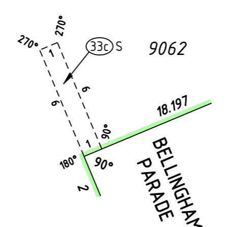
ENLARGEMENT 'L2' SCALE 1:200
