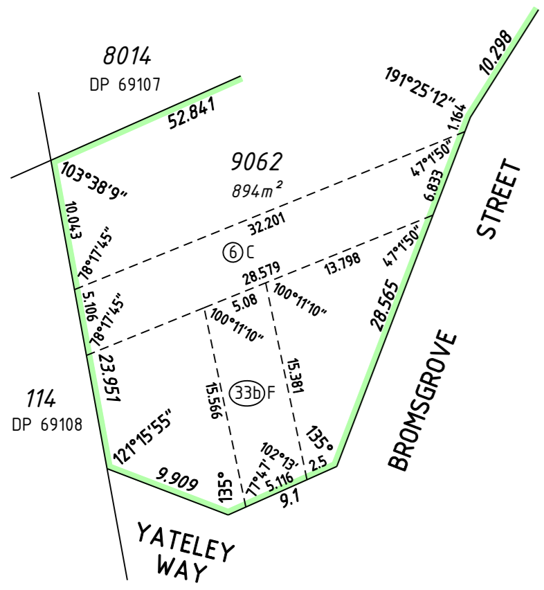
ENLARGEMENT 'F' SCALE 1:400
